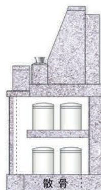
▲納骨棺断面図
